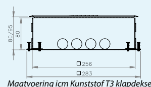
Maatvoering icm Kunststof T3 klapdeksel
